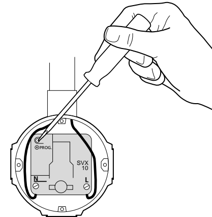
Figuur 2. Activeren en opheffen van de programmeerstand.
