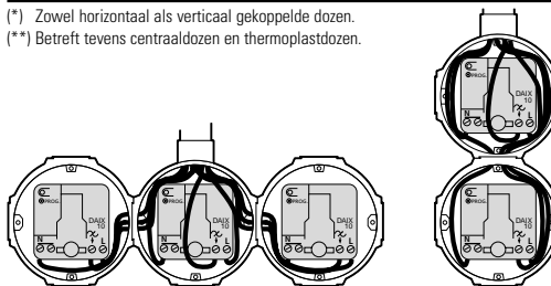
Meervoudige horizontale en verticale inbouwdozen.
